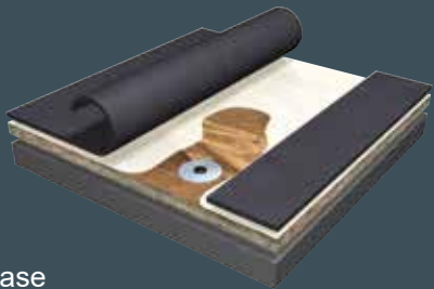
EPDM Totalmente adherido con adhesivo a base de disolvente
