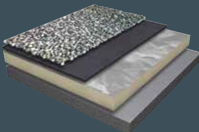
EPDM Lastrado
