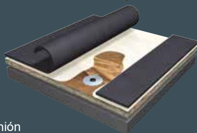
EPDM Totalmente adherido con adhesivo a base de solvente
