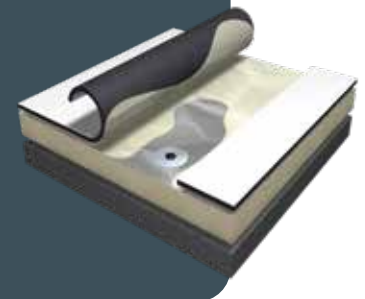
EPDM Totalmente adherido con adhesivo de unión a base de agua
