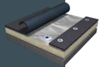
EPDM Conectado mecánicamente
