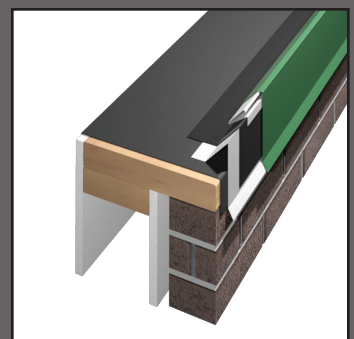
Compresión a presión de 2 piezas
