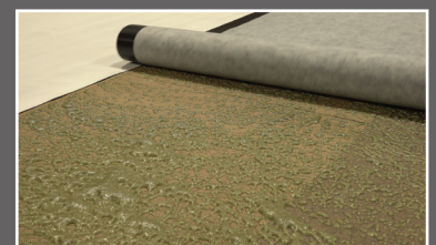
Adherencia de vellón TPO a la salpicadura de hélice.
