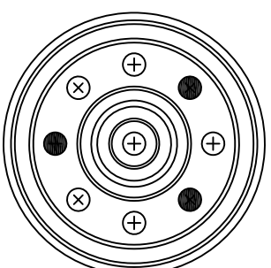
3 FASTENERS PER PLATE
