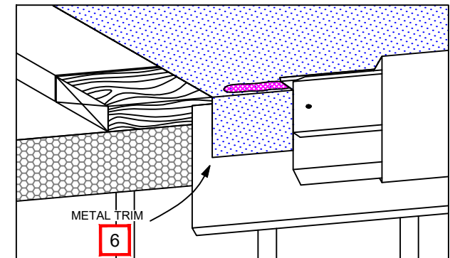
OPTION C - FASCIA EDGE METAL 4
