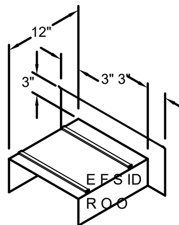
VERSIÓN DE PLACA DE EMPALME DE TAPAJUNTAS EN LA PARED FINAL (SE MUESTRA A LA DERECHA) (DISPONIBLE SOLO EN .040\"/>
