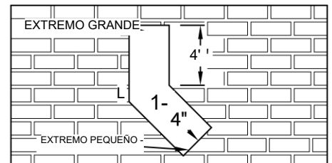
BAJANTE ESTILO B
