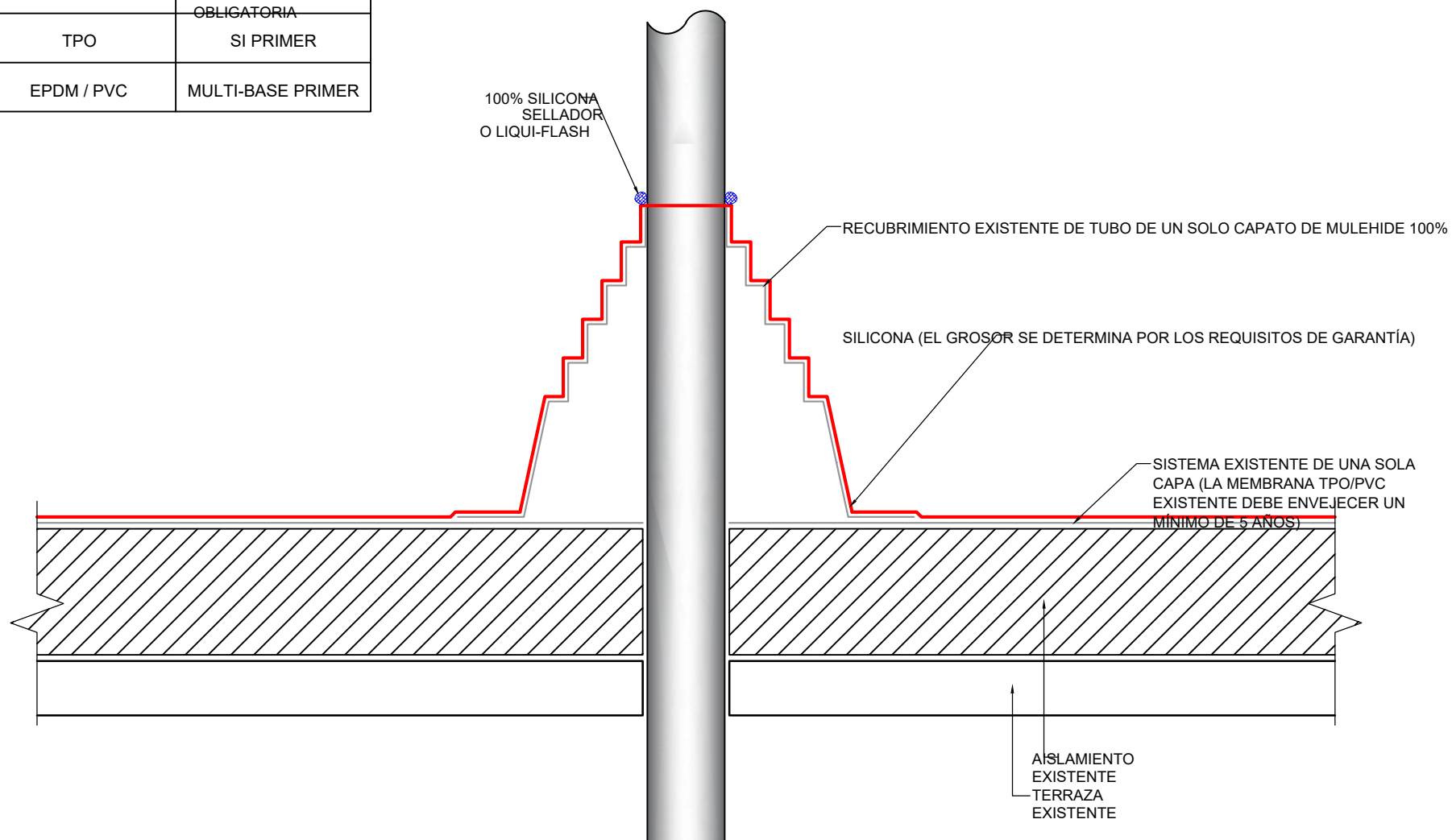
SISTEMAS APLICABLES (Y MEMBRANAS) CONJUNTO MONOCAPA EXISTENTE
